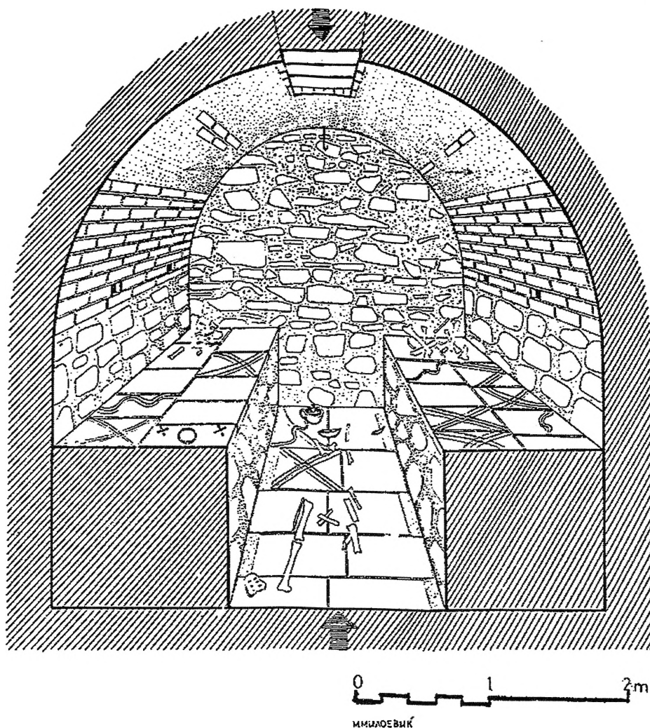
Сл. 2. Пресек на гробницата
