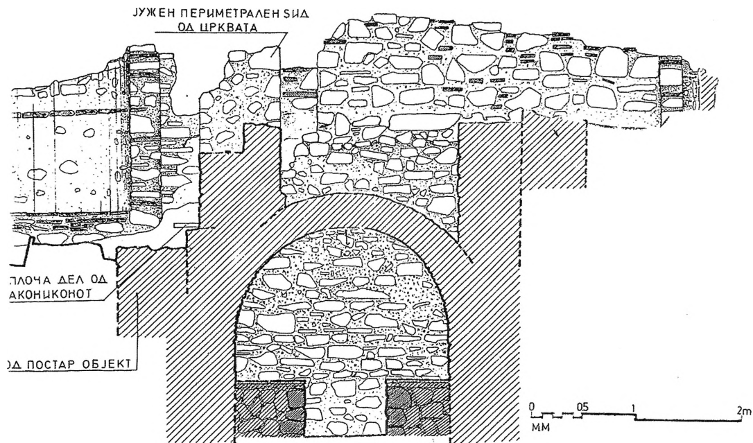
Сл. 4. Пресек на гробницата со придружниот архитектонски објект
